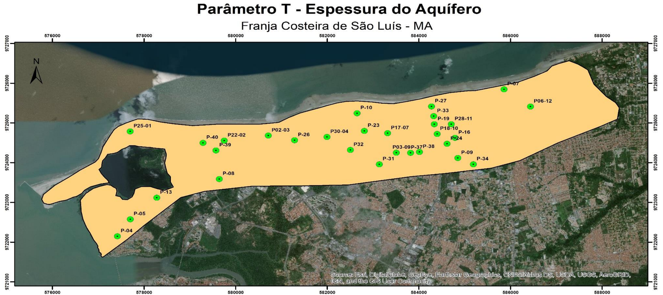
Figura 18: Espessura do aquífero - Parâmetro T - Franja costeira de São Luís – MA
