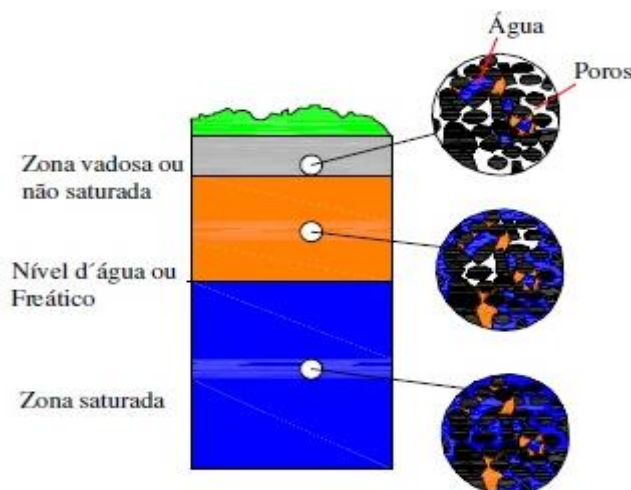
Figura 12: Distribuição de água no subsolo.
