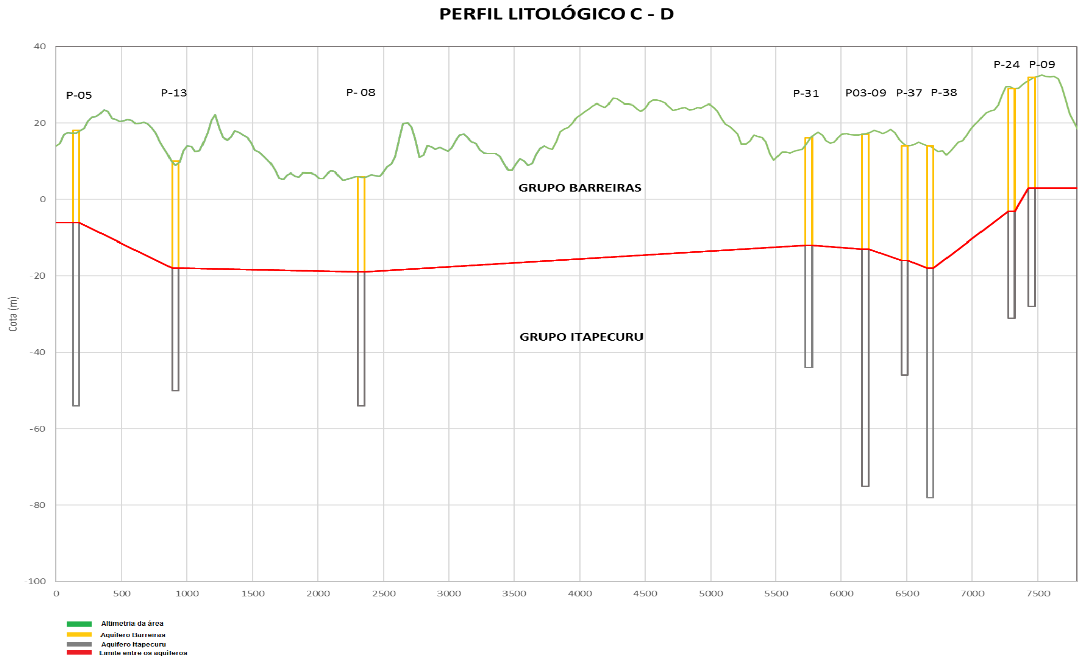
Figura 10: Perfil litológico C - D Figura 17: Perfil litológico C -D dos poços na franja costeira de São Luís – MA
