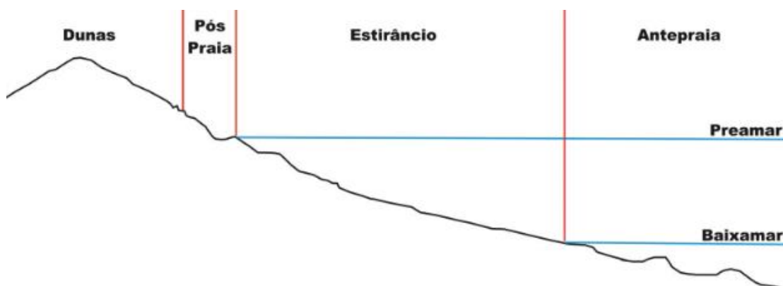
Figura 3: Perfil das praias da área de estudo - Franja costeira de São Luís – MA.
