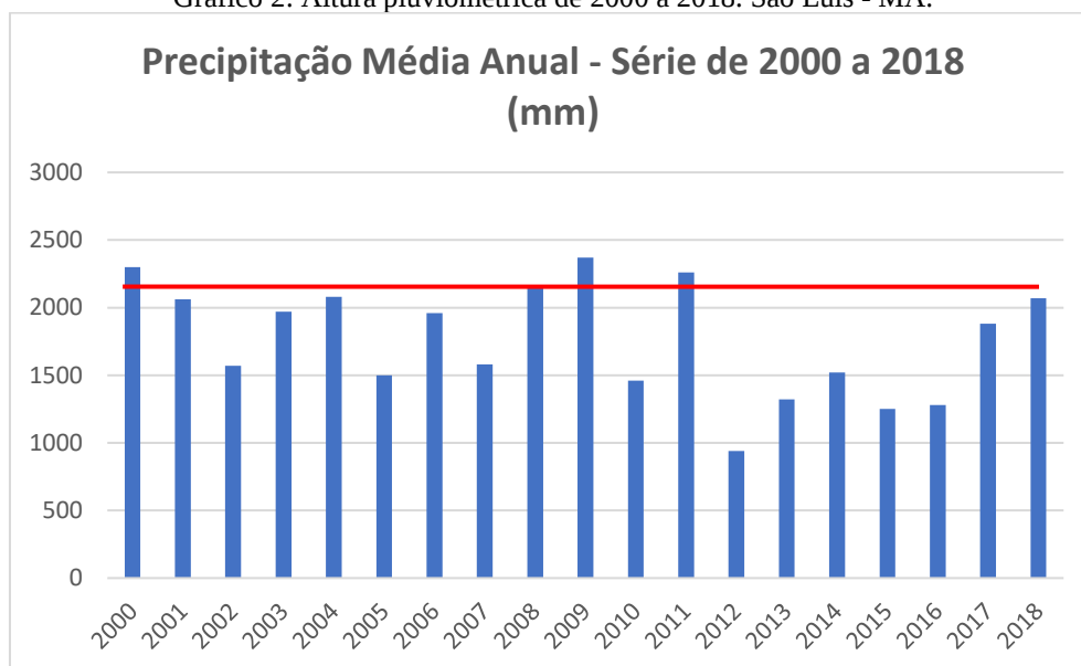
Gráfico 2: Altura pluviométrica de 2000 a 2018. São Luís - MA.
