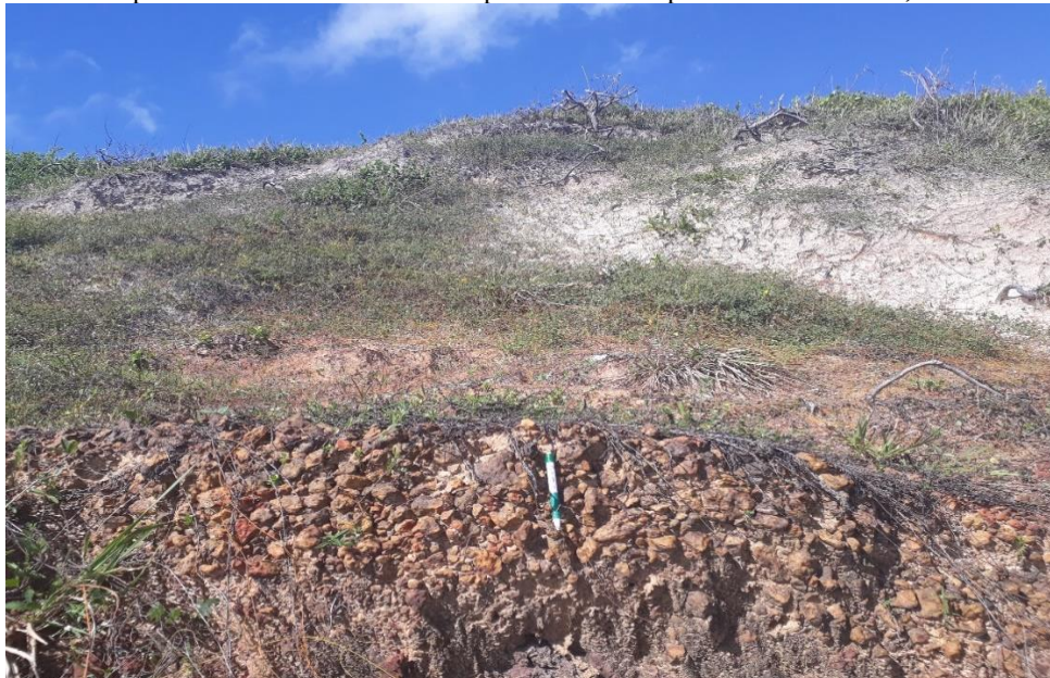
Foto 12: Vista parcial do afloramento do Grupo Barreiras na praia de São Marcos, São Luís – MA.
