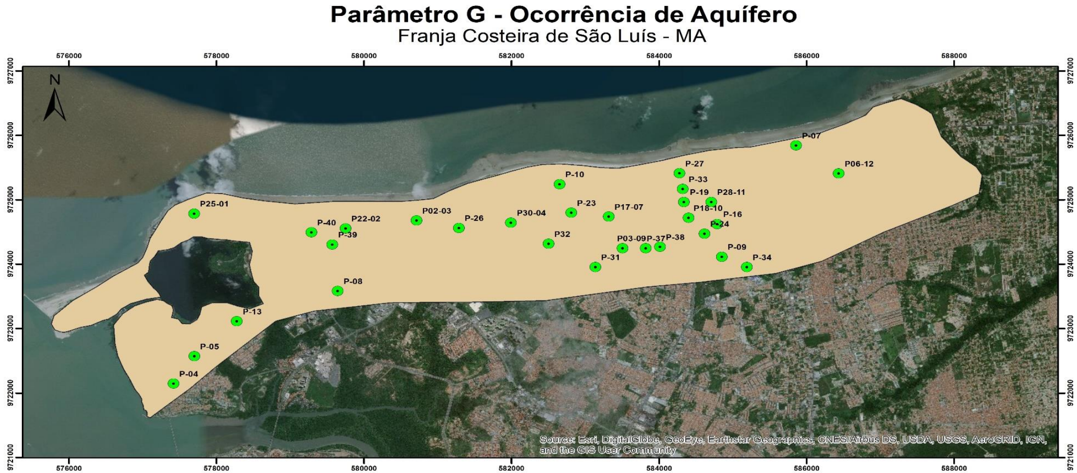
Figura 13: Ocorrência de aquífero – Parâmetro
