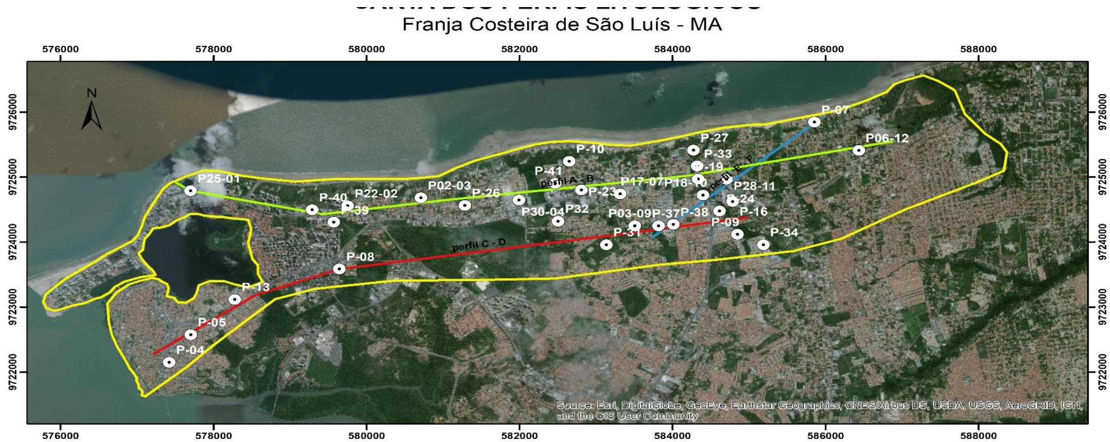
Figura 8: Carta dos perfis litológicos - Franja Costeira - São Luís - MA
