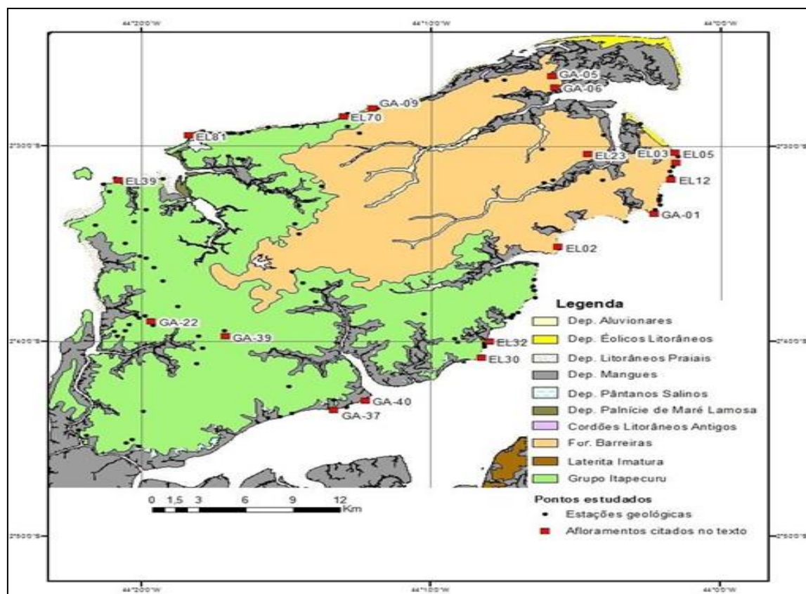
Figura 6: Carta geológica da Ilha do Maranhão.
