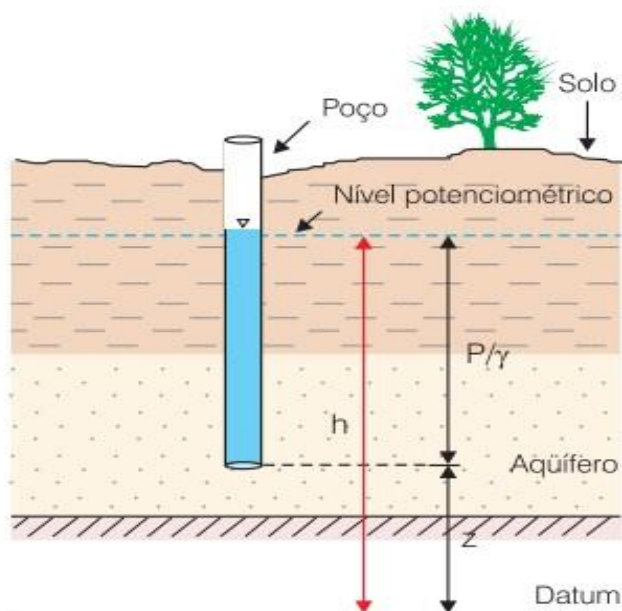
Figura 7: Carga hidráulica em um ponto do aquífero expressa pelo nível piezométrico
